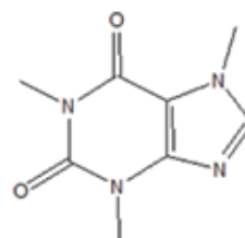
кофеин
