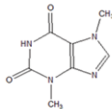
теобромин
